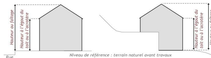
Schéma illustratif - mesures hauteurs des constructions
